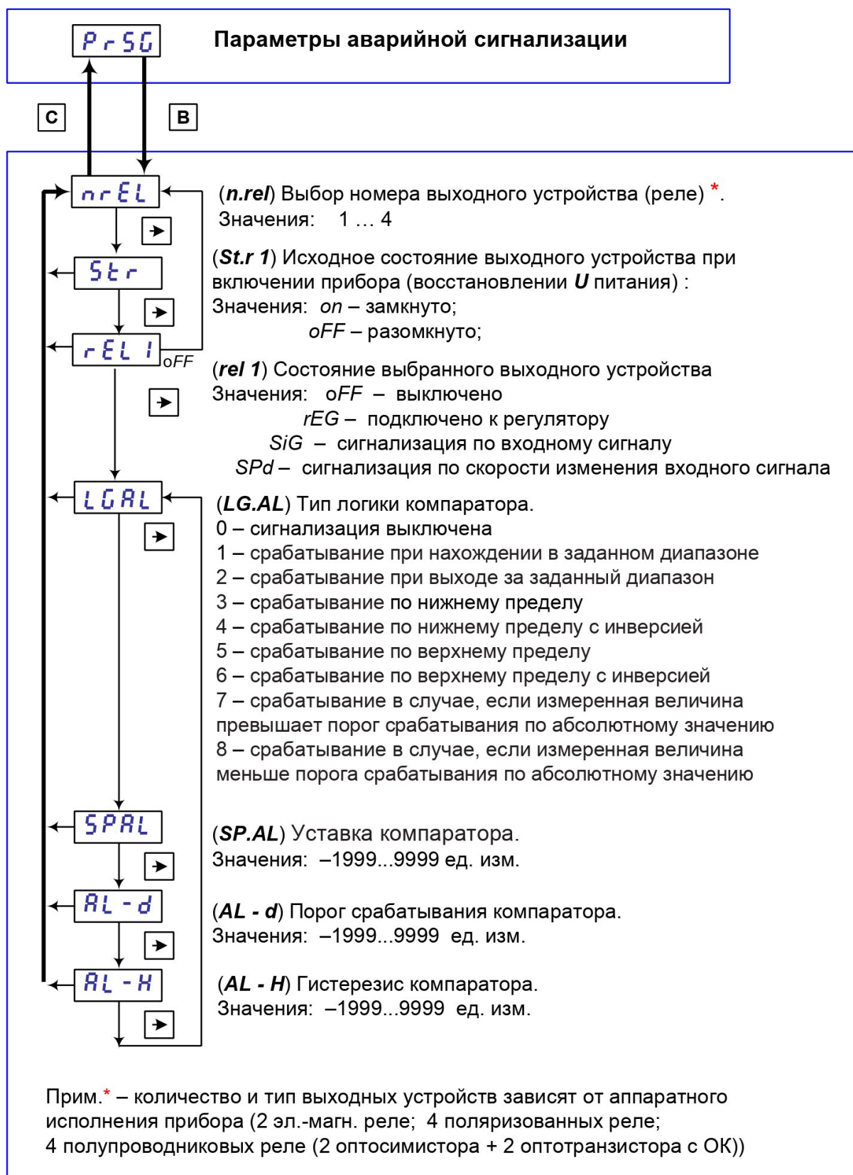
Рисунок 32 – Схема задания параметров аварийной сигнализации.
