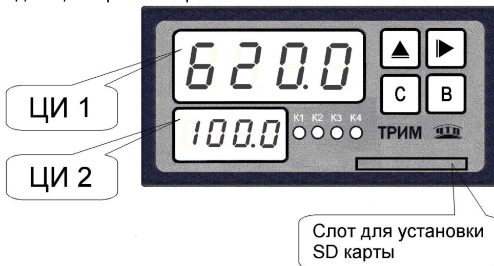
Рисунок 22 – Вид прибора со стороны фронтальной панели.
