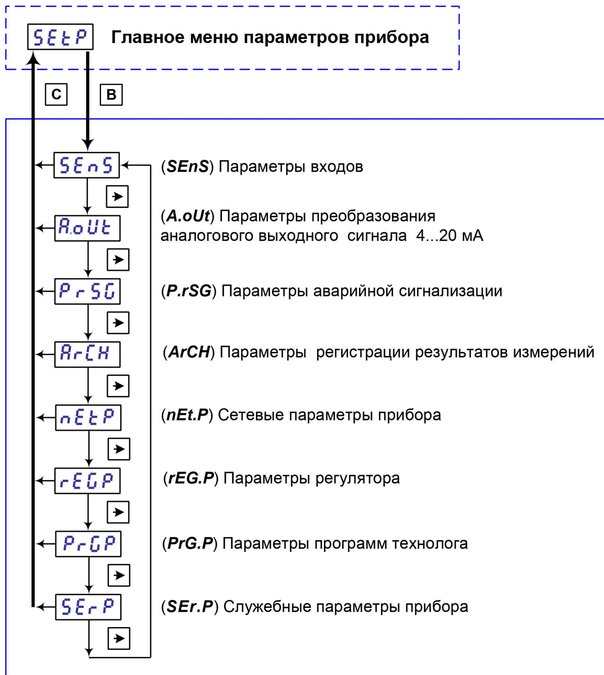
Рисунок 27 – Схема выбора групп рабочих параметров прибора.
