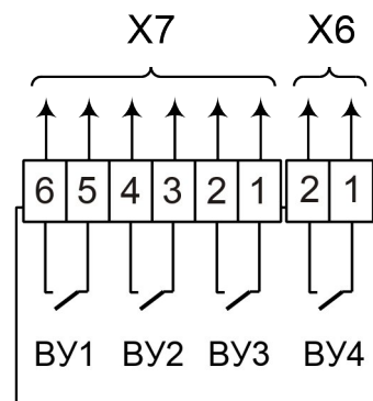
Схема подключения ВУ для исполнений X3X
