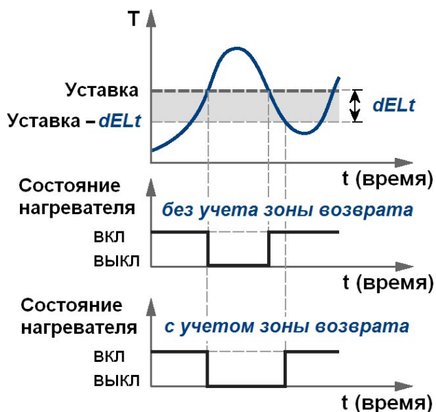
Рисунок 8 – Принцип работы двухпозиционного регулятора
