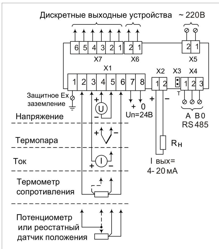
Рисунок Б.1 - Общая схема подключения прибора
