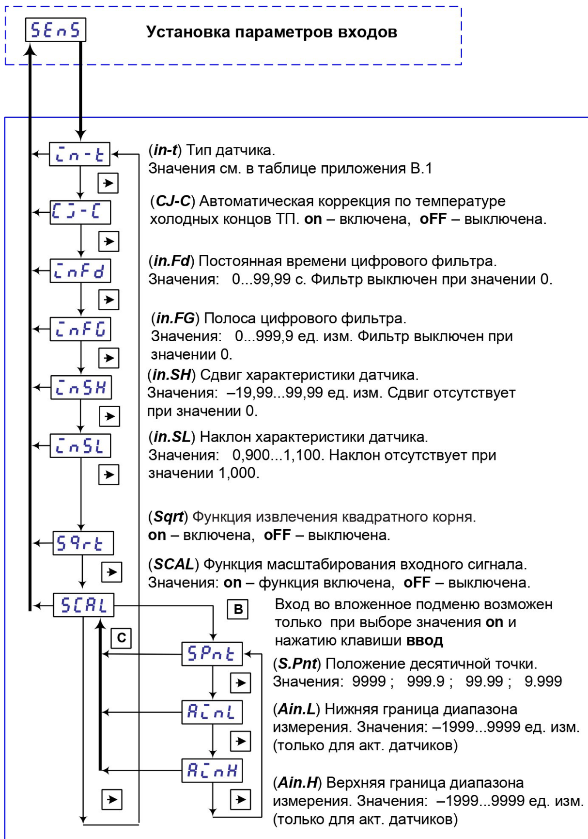
Рисунок 28 – Схема задания параметров входов.
