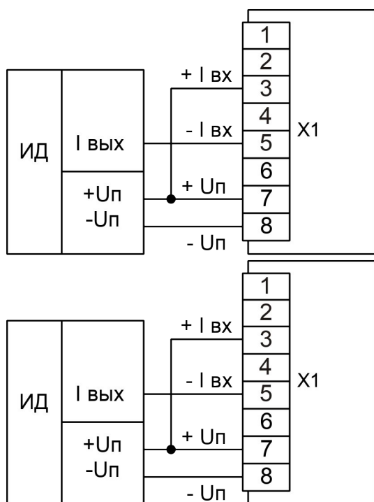
Рисунок 14 – Подключение активных датчиков, с унифицированными выходными сигналами тока, имеющих отдельные цепи питания и трехпроводную схему соединения (например ТСМУ, ТСПУ).
